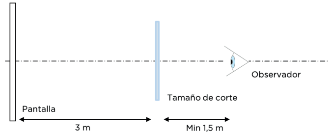
Figura 2: Condiciones de observación estándar de la gama MIRASTAR® para la localización de defectos puntuales.
