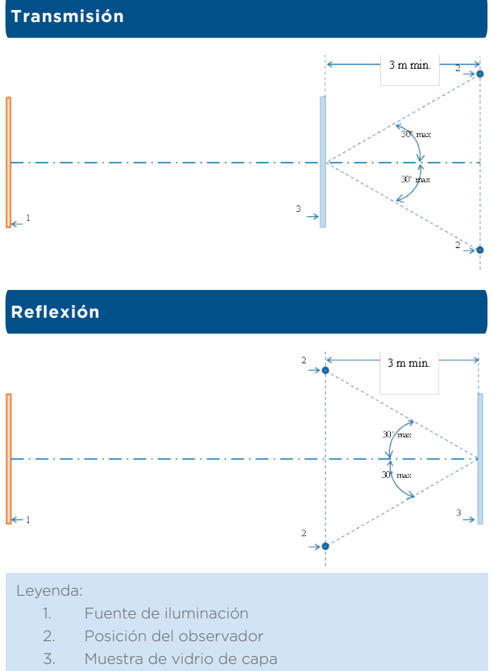
Figura 1: Esquema de los procedimientos de examen del vidrio de capa (según EN 1096-1)
